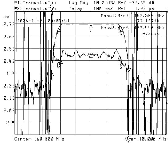
Horizontal: 1.0MHz/Div Vertical: 100nsec/Div&10dB/Div
