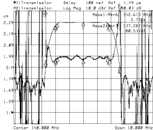
Horizontal: 1.0MHz/Div Vertical: 100nsec/Div&10dB/Div
